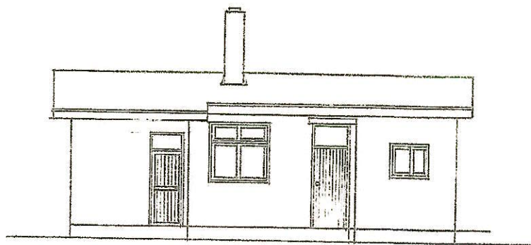
榮町掛水砂地住宅1号 立面图 5-1:100
